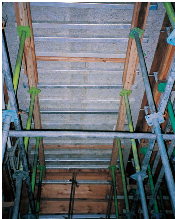
型枠用木毛セメント板を使用した例
